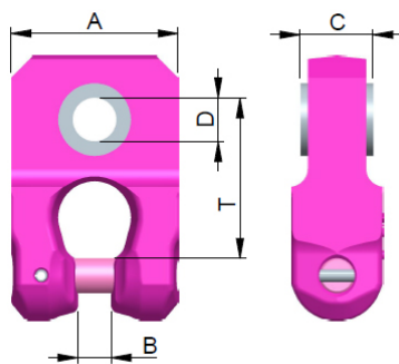
Abb. 2: Isolierlasche V-GIL
